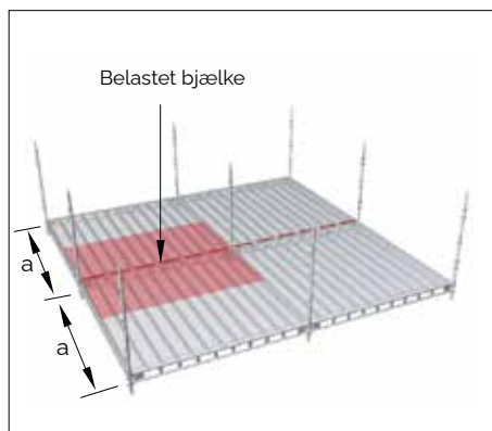
Udvidet stillads
