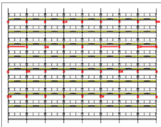
Staging med momenthegn SKRD og forankring
