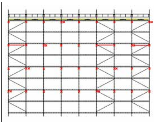
Staging med vertikale diagonalstag og forankring
