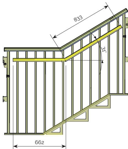
8000055, Gelænder-0.5 m trappeløb, 4.7 kg
