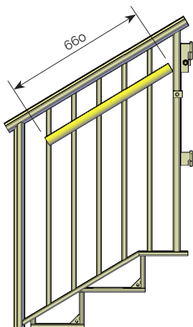
8000050, Gelænder-indgang, 2,2 kg
