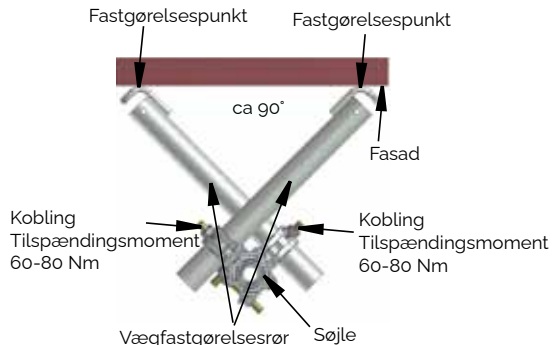
Eksempel på forankring som kan optage horisontalkræfter
